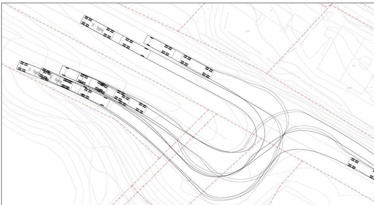
Figur 6: Sporing for vogntog 22 meter (tømmerbil) i krysset
